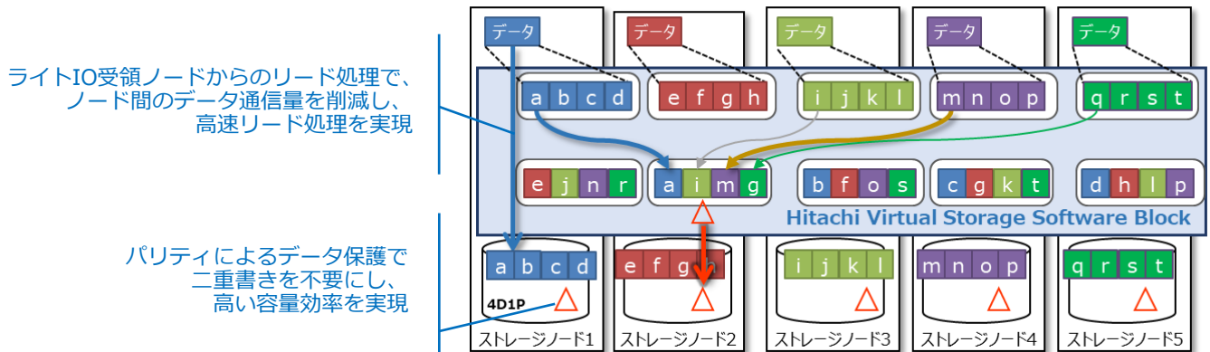
日立独自のデータ保護技術(HPEC 4D+1P*2構成の場合)
